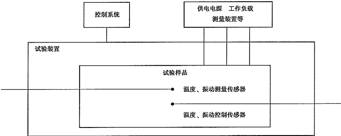
图 1 试验平台示意图
