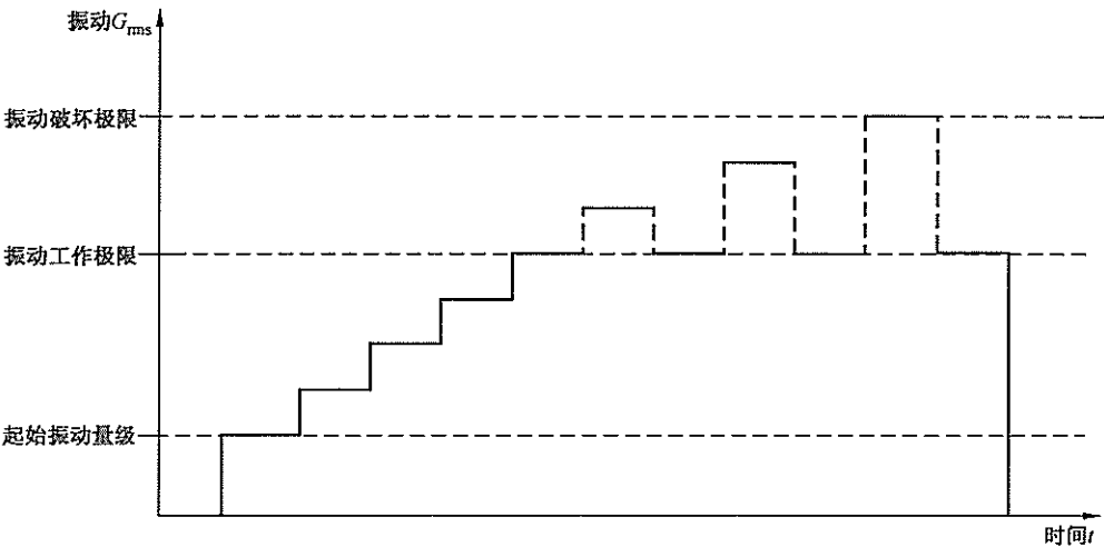
图 5 振动步进试验曲线示意图
