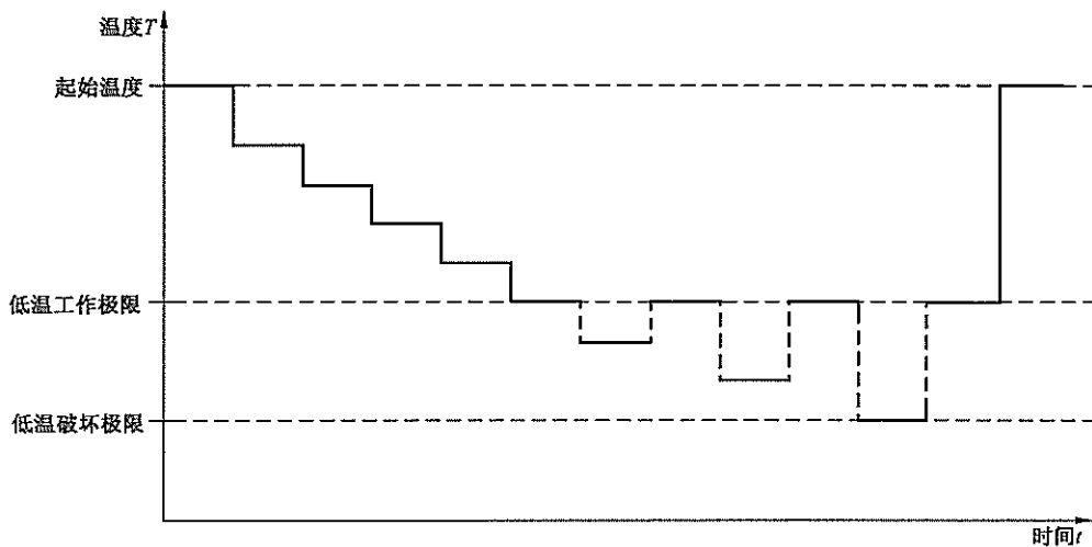
图 2 低温步进试验曲线示意图
